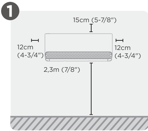
Επιλέξτε τοποθεσία εγκατάστασης
