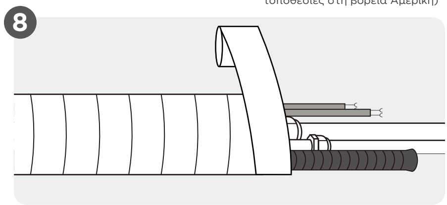
Τυλίξτε σωληνώσεις και καλώδιο (Δεν ισχύει για ορισμένες τοποθεσίες στη βόρεια Αμερική)
