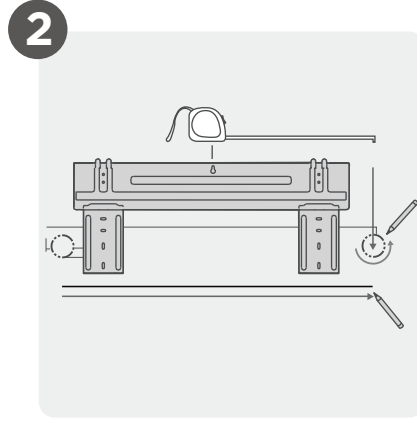
Συνδέστε την πλάκα στήριξης
